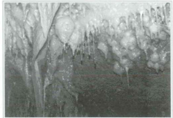
Foto 5. Formaciones estalagtitas con base globular. Sima de la Toba. Foto: Antonio Gil.
